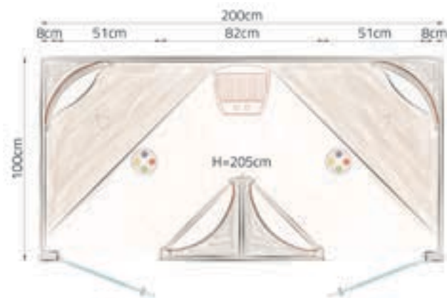
Grundriss-Abbildung Saunaofen-Paket strichliert
